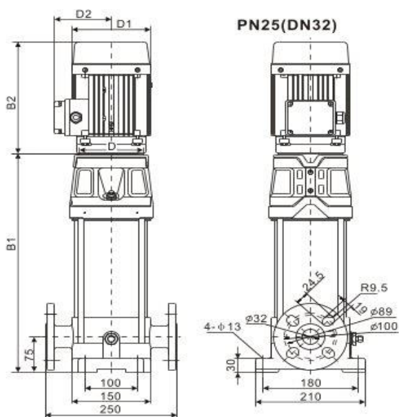
Размеры, мм
