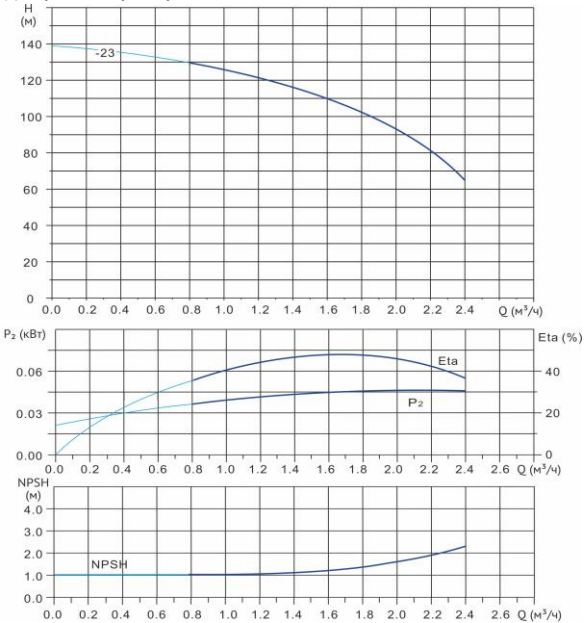
Диаграмма характеристик
