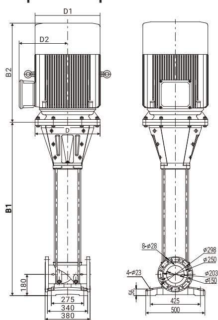
Габаритный чертеж
