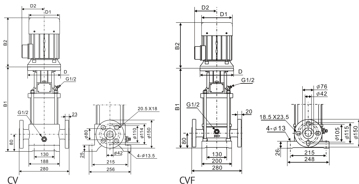
Габаритный чертеж
