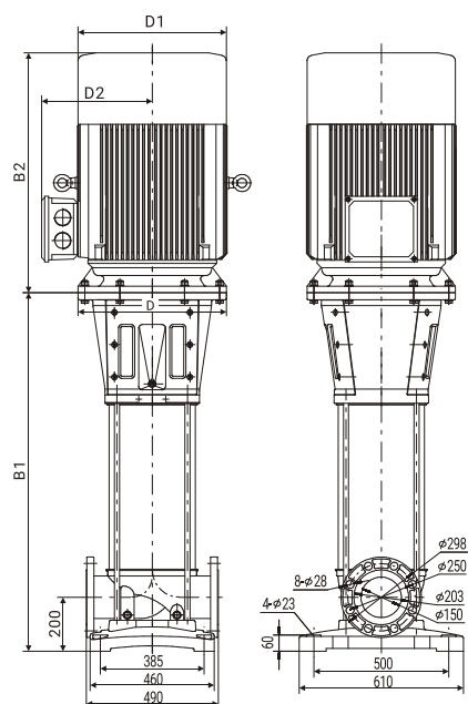
Габаритный чертеж
