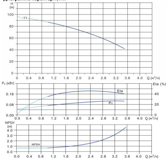
Диаграмма характеристик
