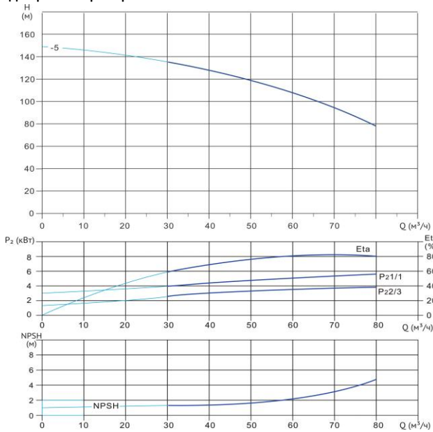
Диаграмма характеристик
