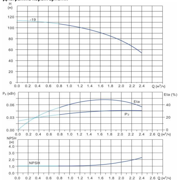
Диаграмма характеристик
