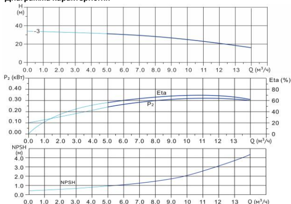
Диаграмма характеристик
