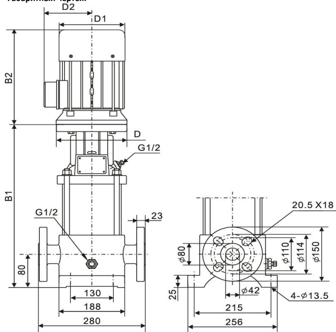
Размеры, мм
