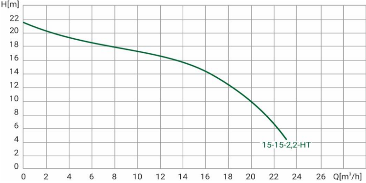
Диаграмма характеристик
