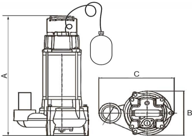
Габаритные размеры
