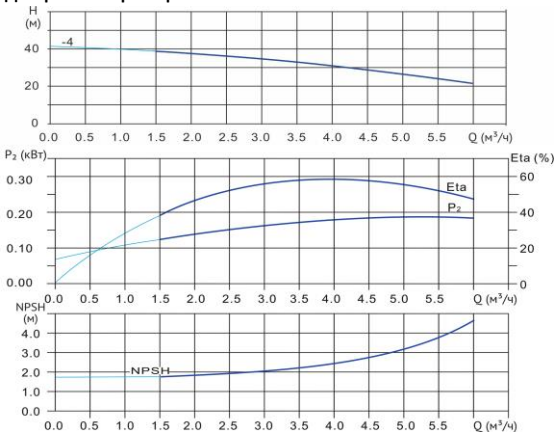
Диаграмма характеристик
