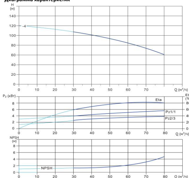
Диаграмма характеристик
