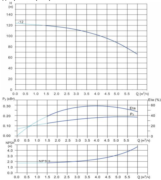
Диаграмма характеристик
