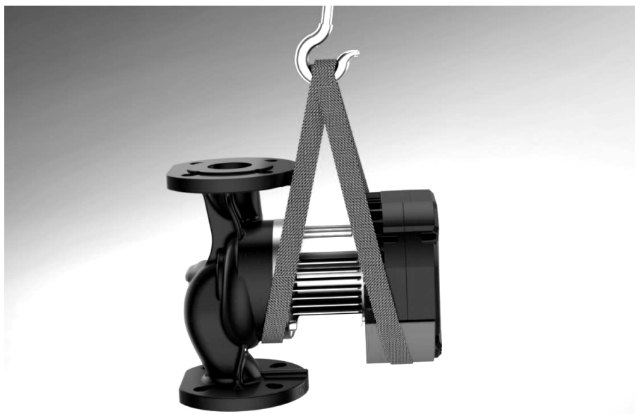
Допустимый способ строповки насоса
