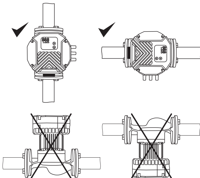
Рисунок 2. Правильное установочное положение насоса отмечено
