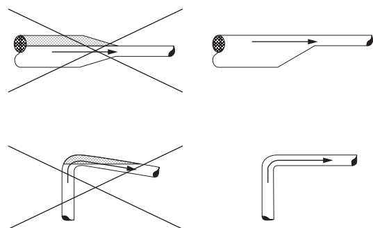
Рисунок 8. Конфигурация трубопроводов на всасывающей стороне.
