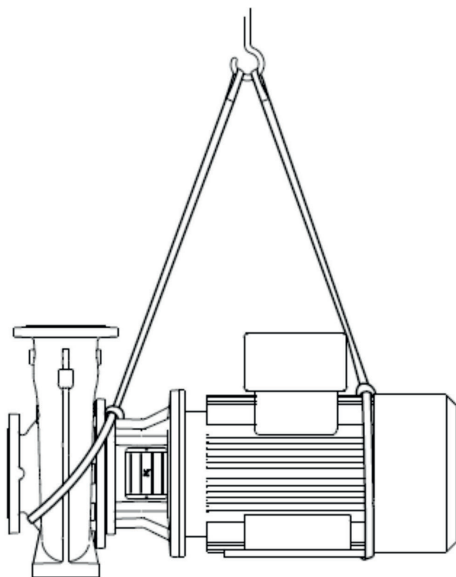
Рис. 1 Правильный способ строповки насоса без плиты-основания
