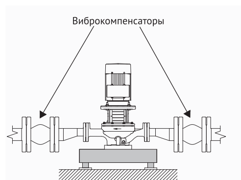
Рисунок 10. Насос TD с виброкомпенсаторами большего диаметра.
