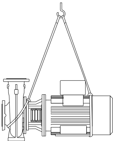
Рис. 1. Правильный способ строповки без плиты-основы
