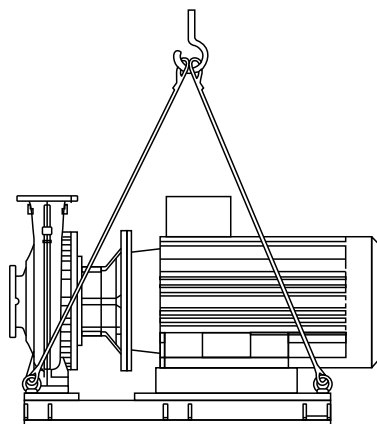
Рис 2. Правильный способ строповки с плитой-основанием
