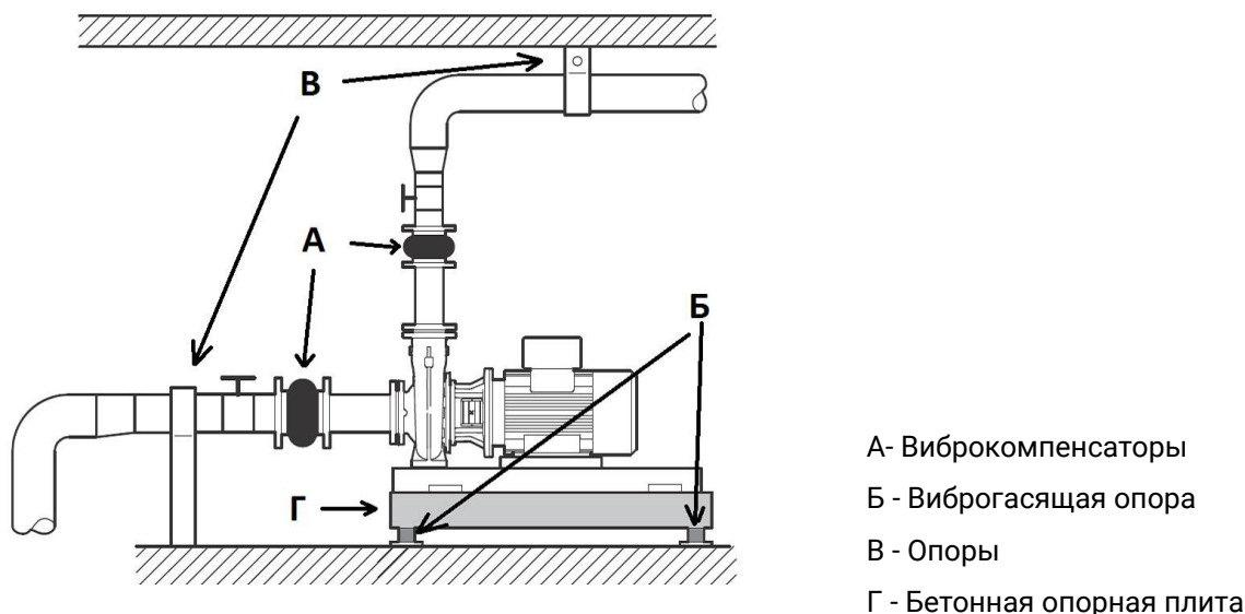
Рис. 7 способы устранения шума и вибраций
