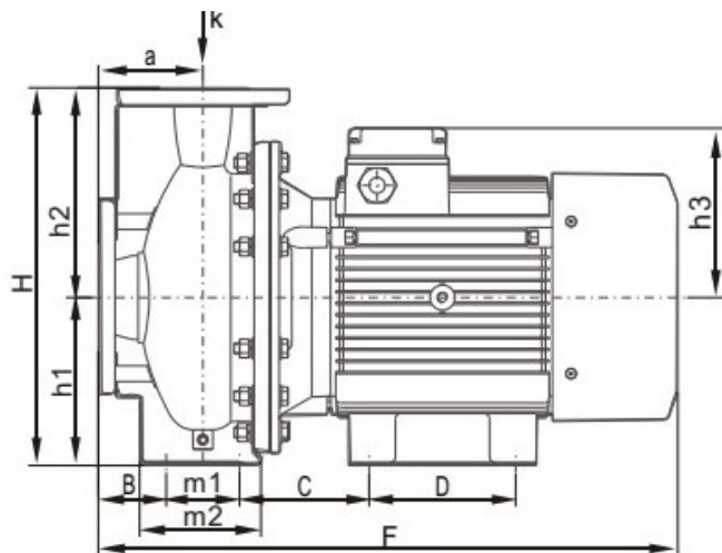
Рисунок.3. Горизонтальный монтаж насоса
