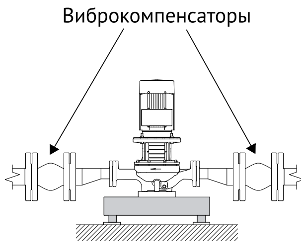
Рис. 8. Насос ТГ с виброкомпенсаторами большего диаметра.
